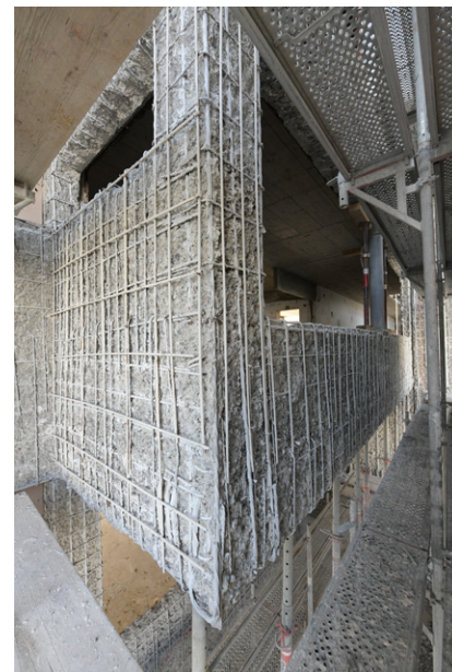
Les façades (2600 m 2 au total) sont assainies avec la technique de l'hydrodémolition (jet à très haute pression) du béton, qui est atteint par le phénomène de carbonatation sur une épaisseur de 4 à 5 cm. Un produit de protection est ensuite appliqué sur l'armature existante pour stopper le phénomène de corrosion, puis l'armature est complétée. Les piliers métalliques trop corrodés sont remplacés.
